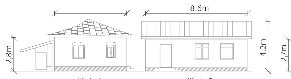
edificio A prospetto nord ovest
